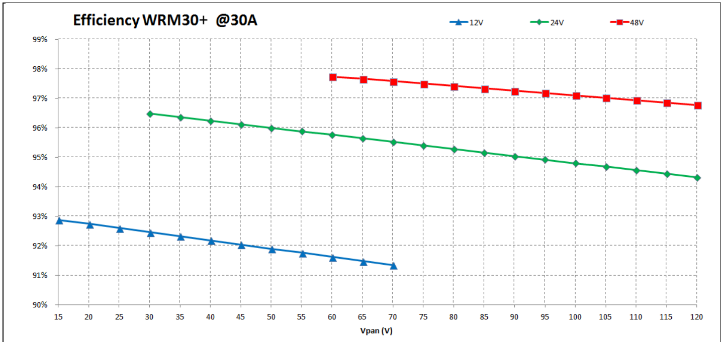
Graf. 2 Eficiencias
