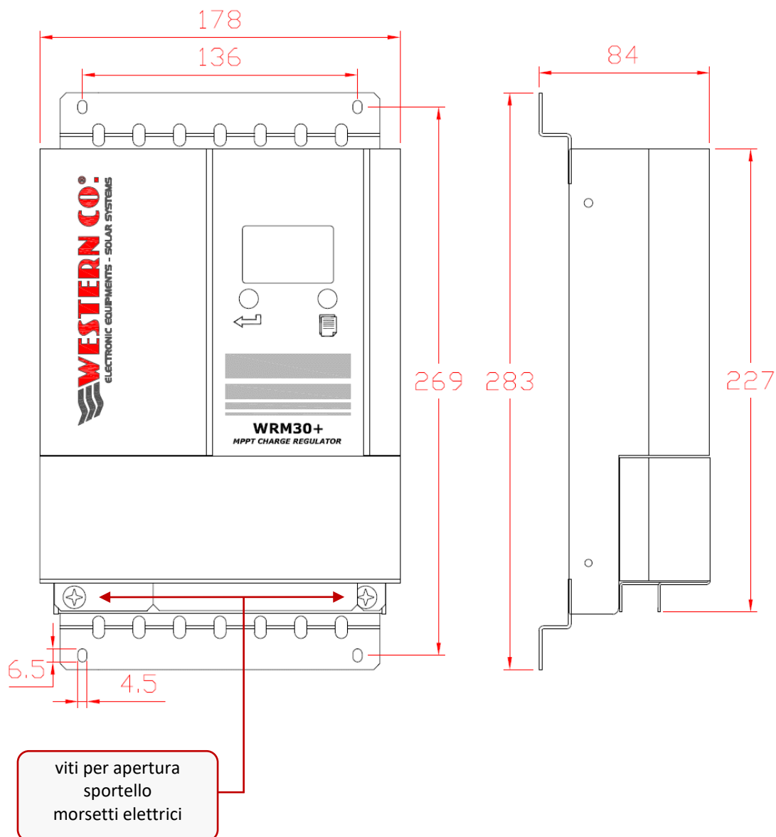
Fig. 4 Dimensioni (mm)
