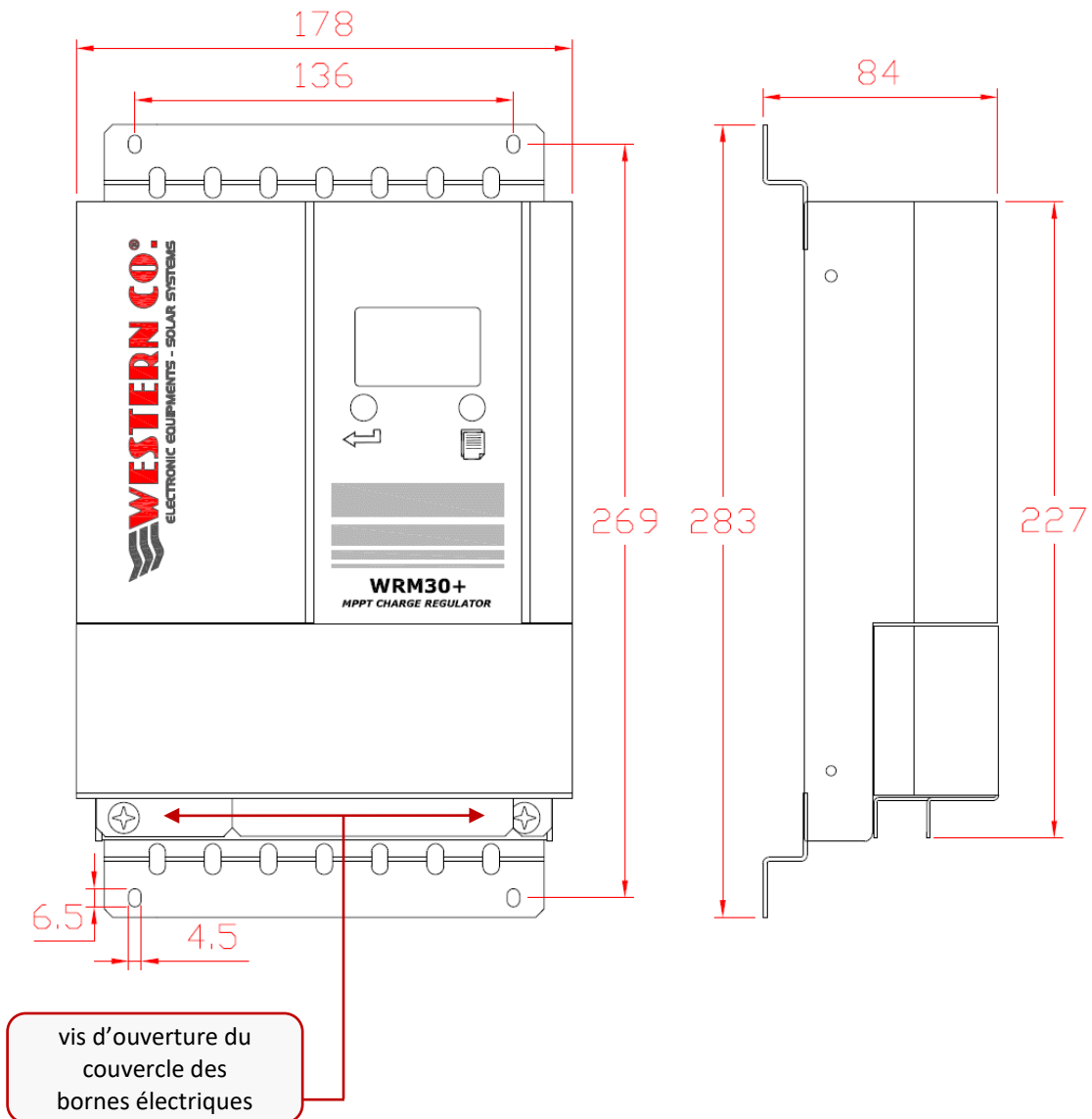
Fig. 4 Dimensions (mm)
