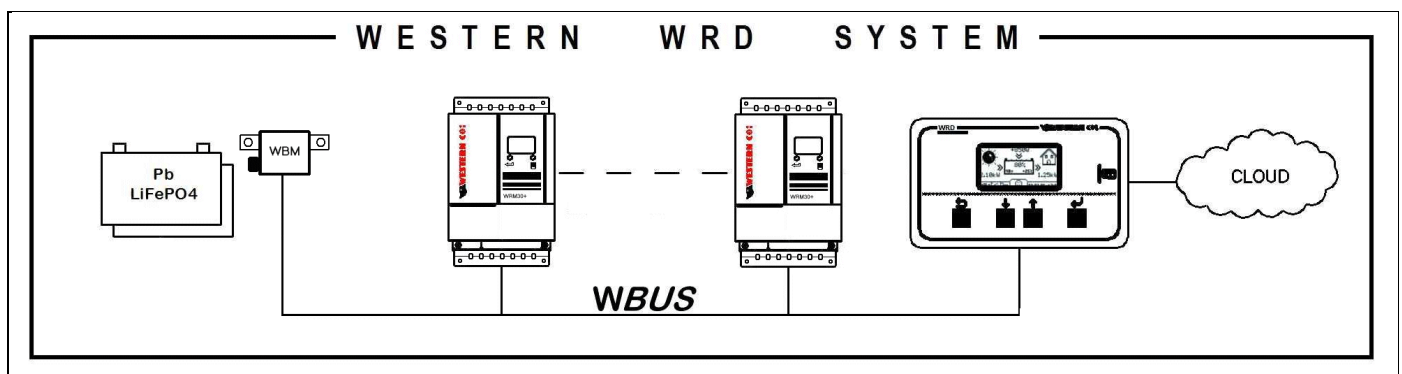
Fig. 3 Esquema de ejemplo del WESTERN WRD SYSTEM
