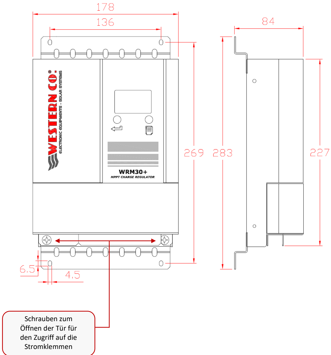
Abb. 4 Ausmaße (mm)
