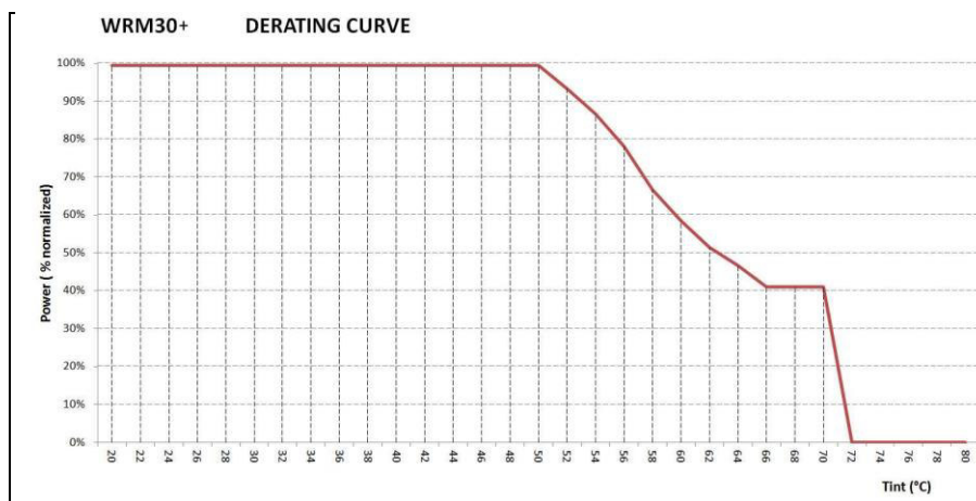
Graf. 3 Derating-Kurve
